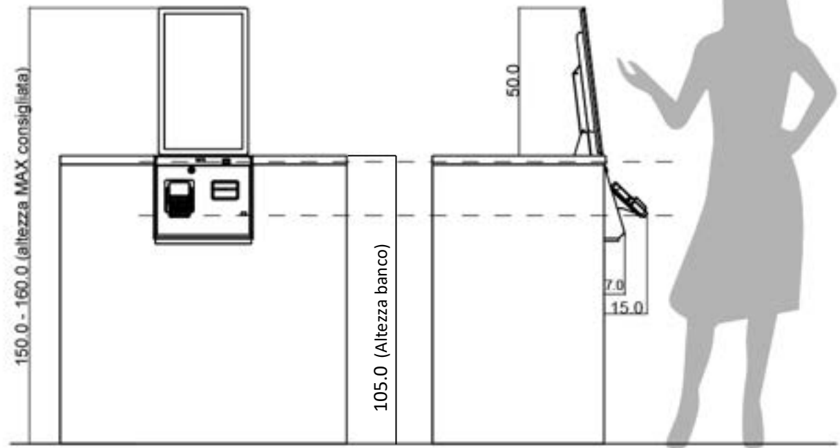
Vista frontale
