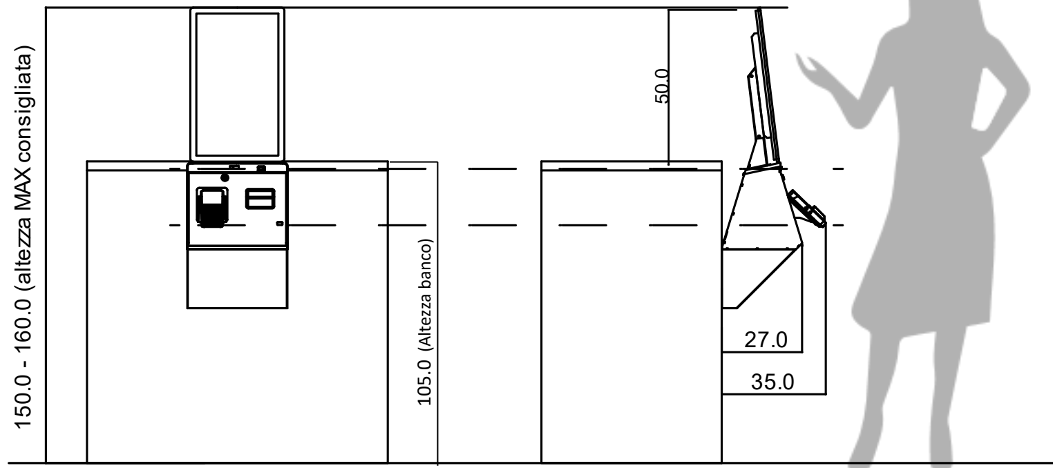
Vista frontale
